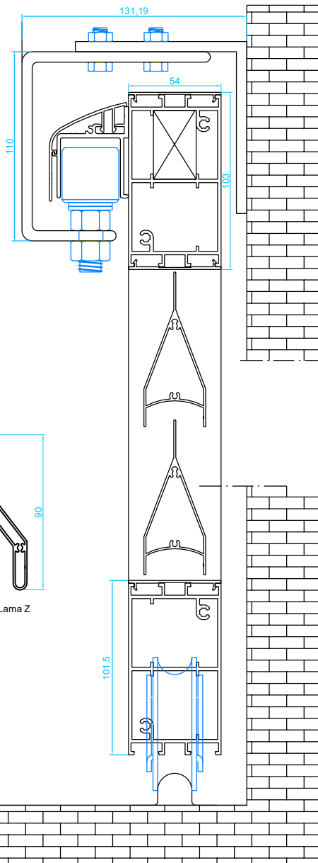
Sección vertical hoja con lamas
