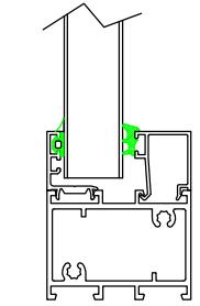
Sección inferior de puerta
