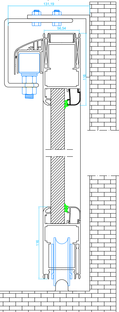
Sección vertical hoja con panel
